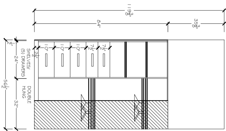
B ELEVATION
